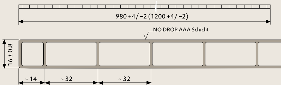
Querschnitt der PLEXIGLAS® Resist AAA SDP 16 (Maße in mm)
