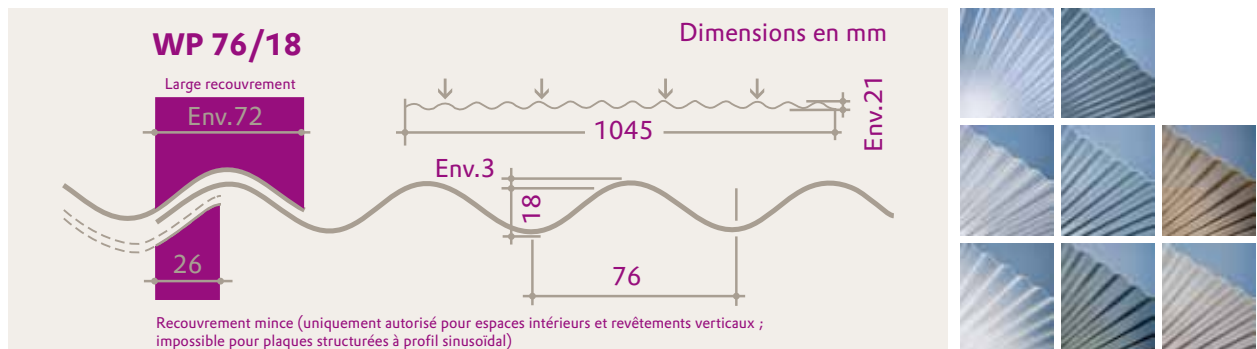
Coupe transversale d'une plaque PLEXIGLAS RESIST® WP 76/18 (dimensions en mm)
