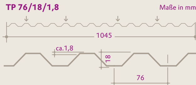
Querschnitt der PLEXIGLAS® Resist TP 76/18/1,8 (Maße in mm)
