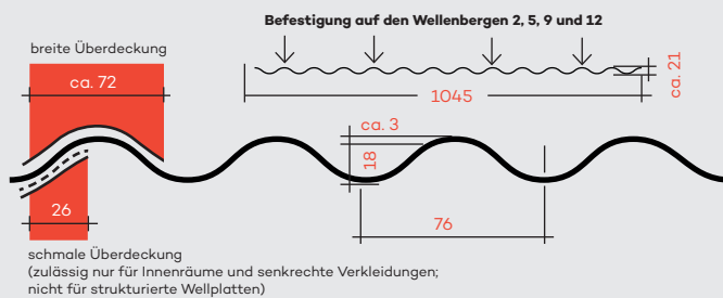
Querschnitt der PLEXIGLAS® Resist WP 76/18/3
