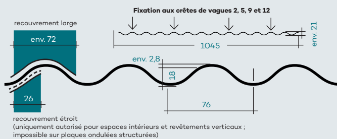
Coupe transversale du PLEXIGLAS® Heatstop Opal WP 76/18/2,8
