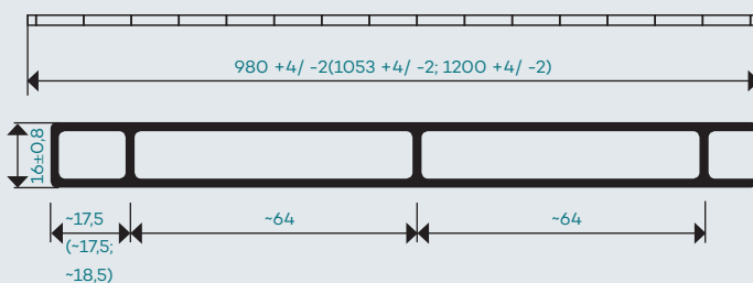
Sección de PLEXIGLAS® Alltop SDP 16 (dimensiones en mm)
