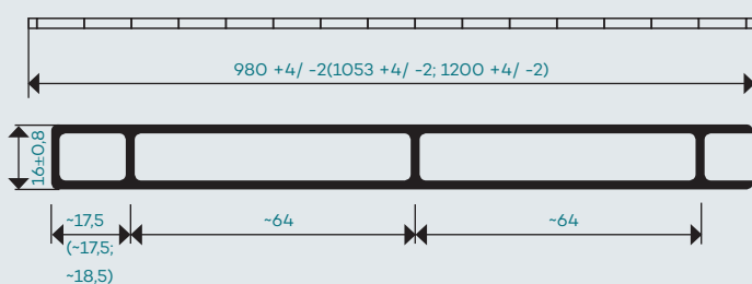
Sezione del PLEXIGLAS® Alltop SDP 16 (misure in mm)
