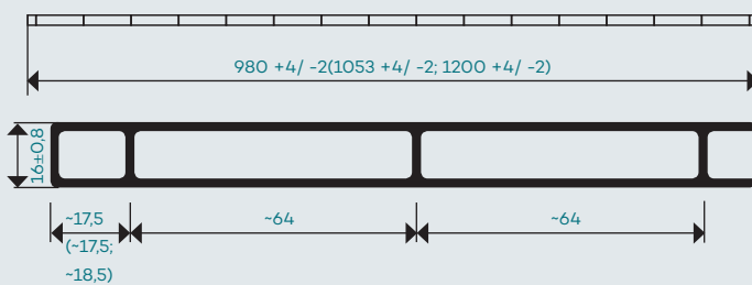
doorsnede van de PLEXIGLAS® Alltop SDP 16 (afmetingen in mm)
