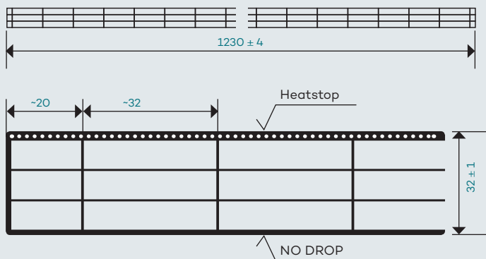
Coupe transversale de la plaque PLEXIGLAS® Heatstop Opal S4P 32 (dimensions en mm)
