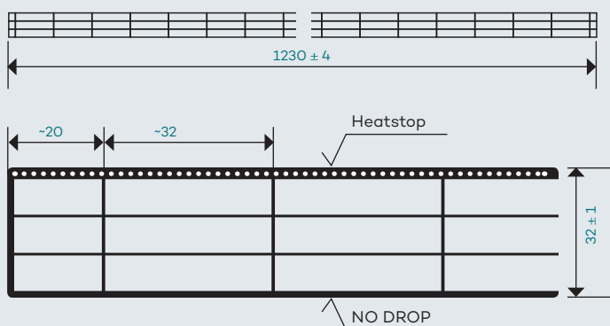
Sezione trasversale PLEXIGLAS® Heatstop Opalescente S4P 32 (dim. in mm)
