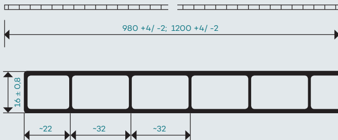
Coupe transversale de la plaque PLEXIGLAS® Heatstop Opal SDP 16 (dimensions en mm)
