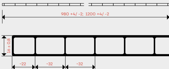
Sezione trasversale di PLEXIGLAS® Heatstop opalescente SDP 16/ (misurata in mm)
