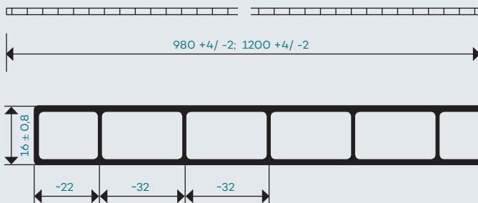
Querschnitt der PLEXIGLAS® Heatstop Cool Blue SDP 16/ (Maße in mm)
