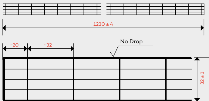
Querschnitt der PLEXIGLAS® Heatstop Cool Blue S5P 32 (Maße in mm)
