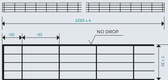
Querschnitt der PLEXIGLAS® Heatstop Opal S5P 32 (Maße in mm)
